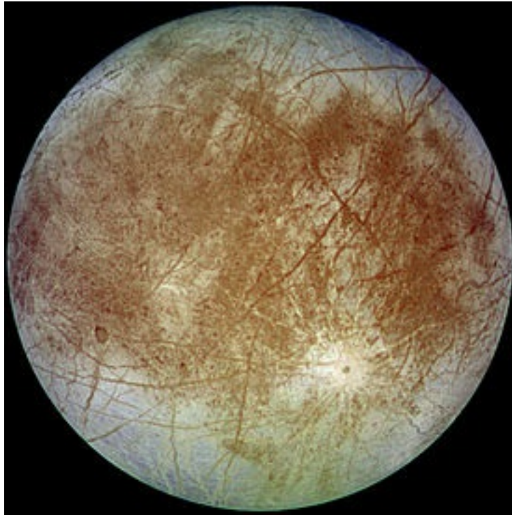
(Europa)
